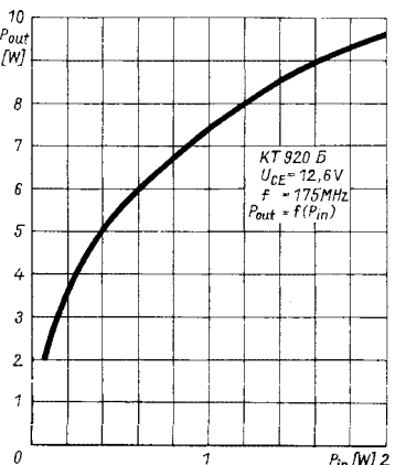
Bild 9: KT 920 B-Ausgangskennlinien
